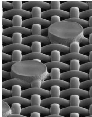
Schablonen-Haftung von SEFAR® PET 1500 120/305-34Y
