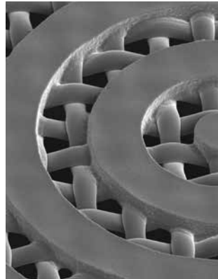
Unterstrahlungsschutz mit SEFAR® PET 1500 120/305-34Y
