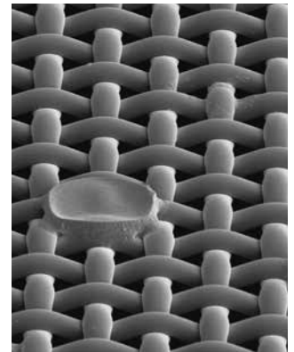
Schablonen-Haftung von Standard Polyestergewebe 120/305-34Y
