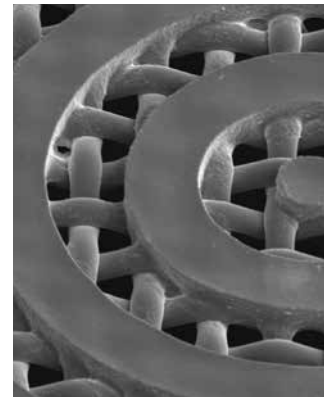
Unterstrahlungsschutz von unbehandeltem Polyestergewebe 120/305-34Y
